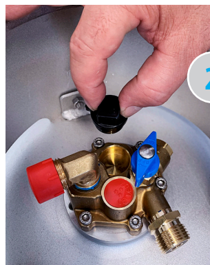
Die alte Anzeigeeinheit durch die Neue ersetzen
