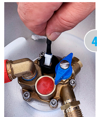
Den Stopfen entfernen und das Kabel des Moduls in den dafür vorgesehenen Platz einstecken
